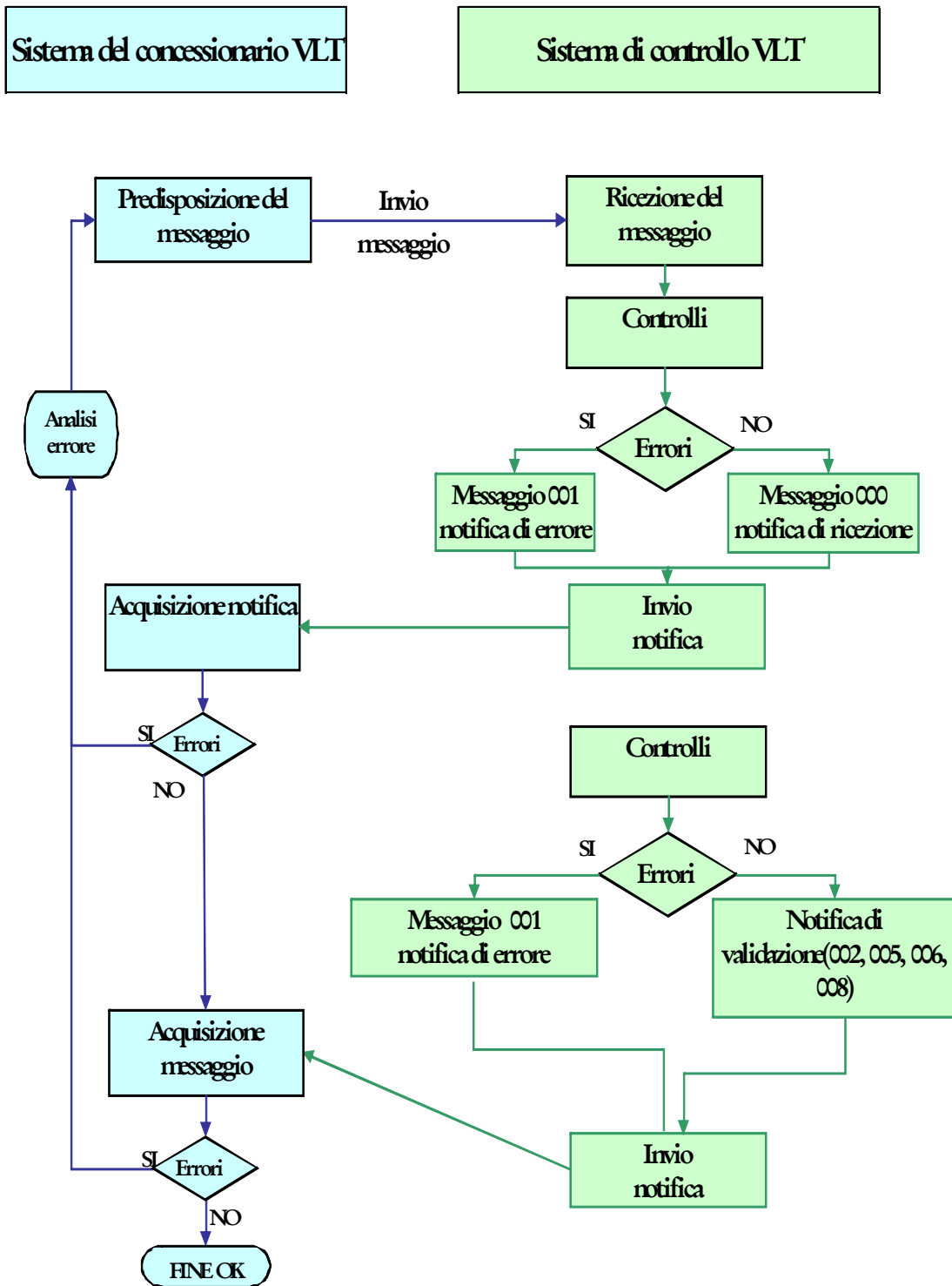
Figura 1 Flusso di comunicazione sistema del concessionario VLT - sistema di controllo VLT
